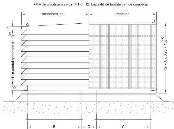
Vooranzicht
