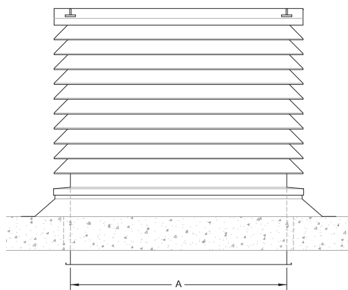
Zijaanzicht Schoepenkap
