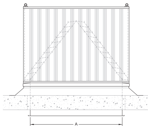
Zijaanzicht Tredekap
